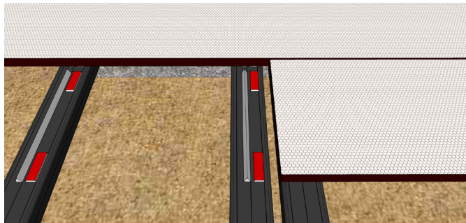
Abb. 5: Doppelte Unterkonstruktion
