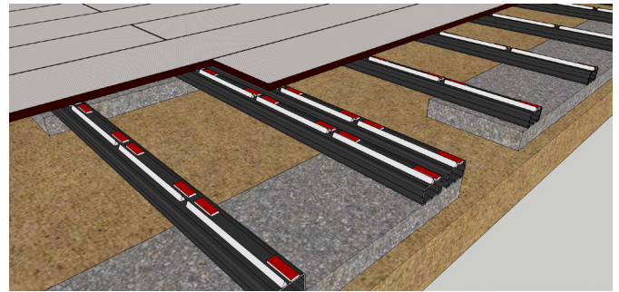
Abb. 6: Montageband und -kleber
