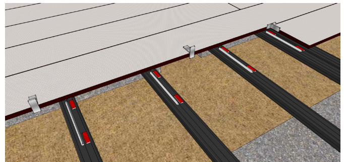
Abb. 7: Aluminium T-Stücke
