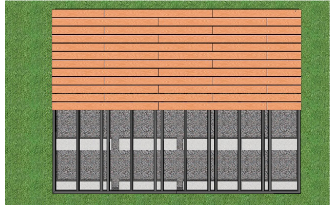
Unterbau, UK und Deck bei 1/2 Längensversatz. Achsmaße: 404-404-117-404-404-117..mm
