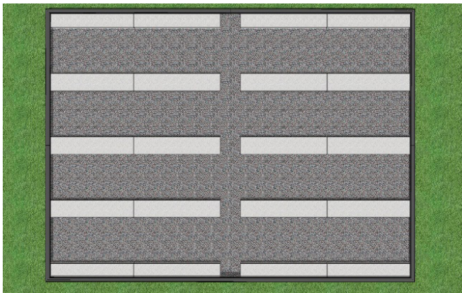
Unterbau, UK und Deck bei 1/2 Längensversatz. Achsmaße: 404-404-117-404-404-117..mm
