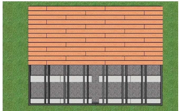
Unterbau, UK und Deck bei 1/3 Längensversatz. Achsmaße: 500-117-500-117-500..mm
